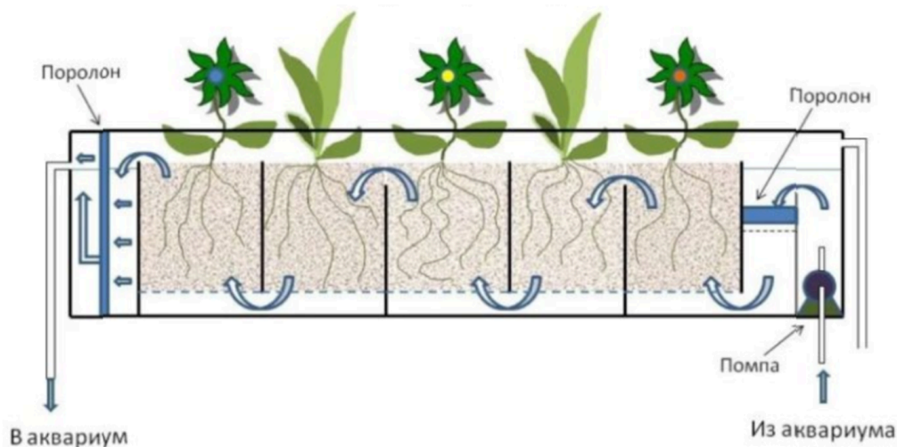
Рис. 2 – Схема фитофильтра
