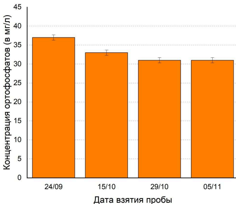
Рис. 6 - График зависимости концентрации фосфатов от времени мониторинга
