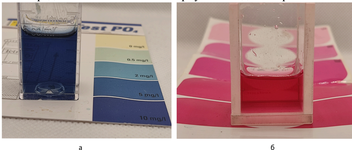
Рис. 5: а - экспресс-тест на фосфаты, б - экспресс-тест на нитраты
